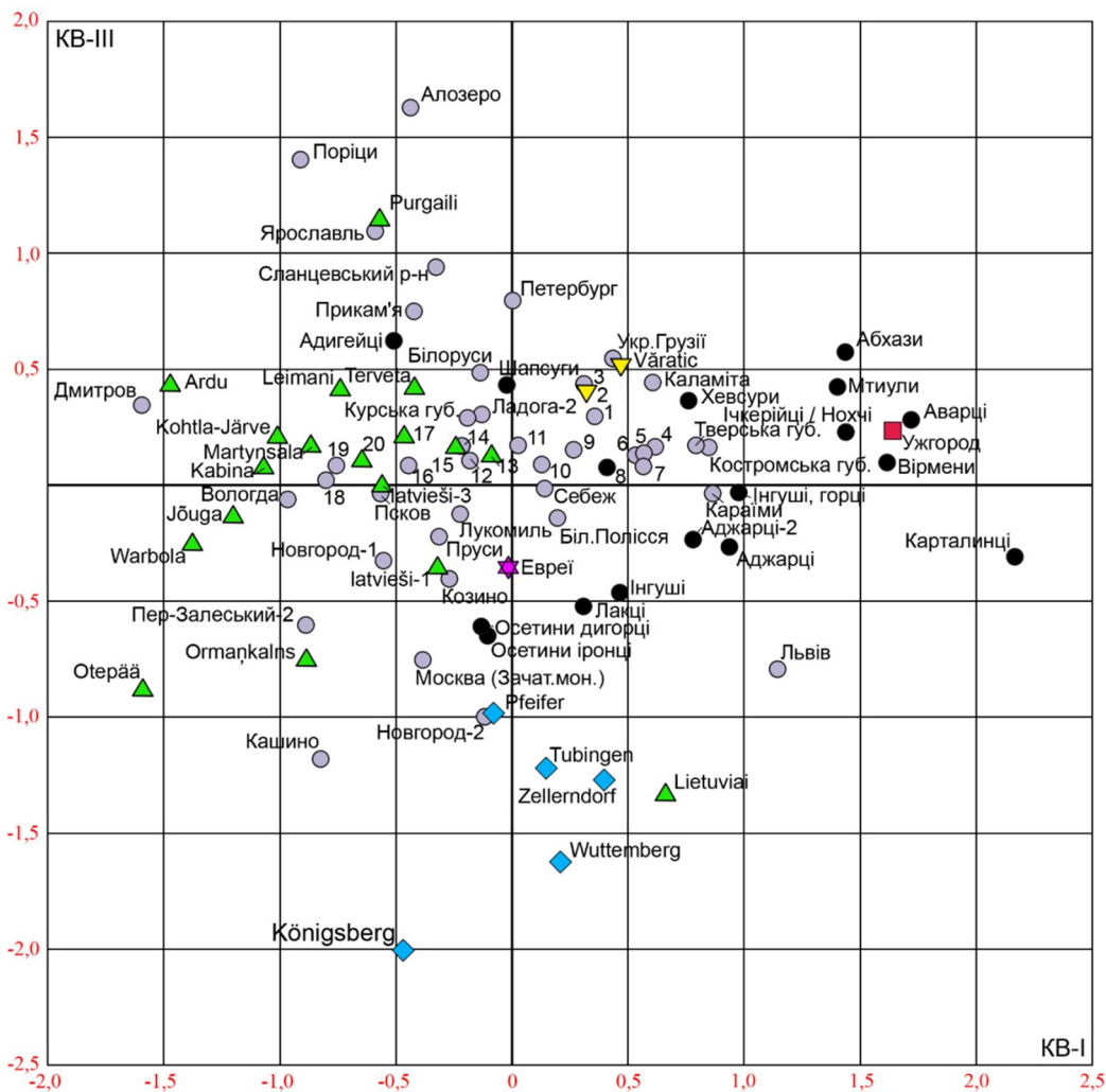
Рис. 4. Розташування 86 чоловічих серій у двовимірному просторі КВ I та КВ III за даними краніометрії.
