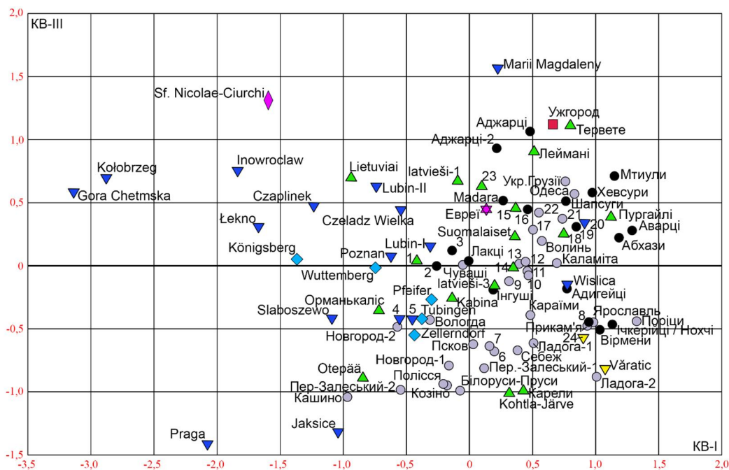
Рис. 7. Розташування 94 чоловічих серій у двовимірному просторі КВ I та КВ III за даними короткої краніологічної програми.
