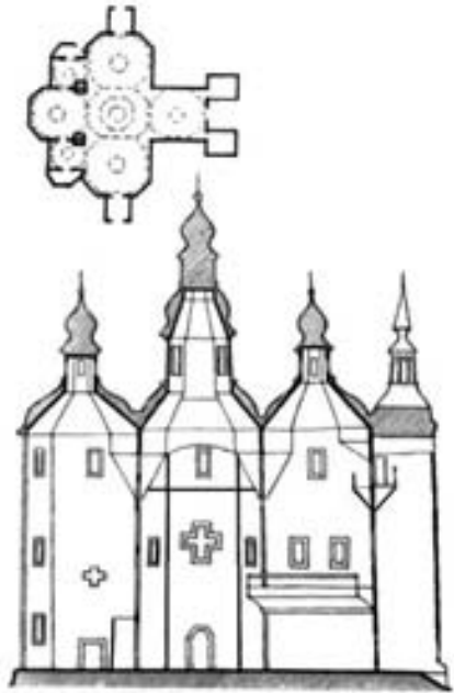
Вознесенська церква в Березні (1761) План і розріз.
